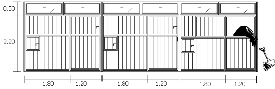
PARETI POSTERIORI
